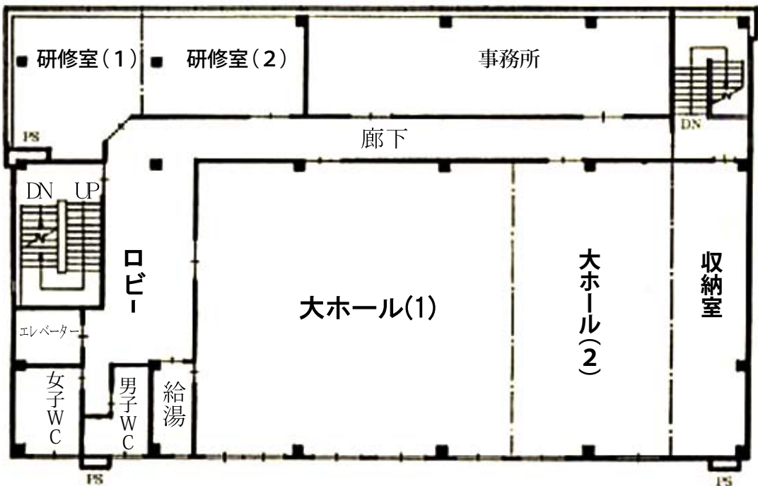
3階 間取図
