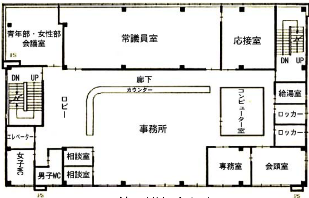
2階 間取図
